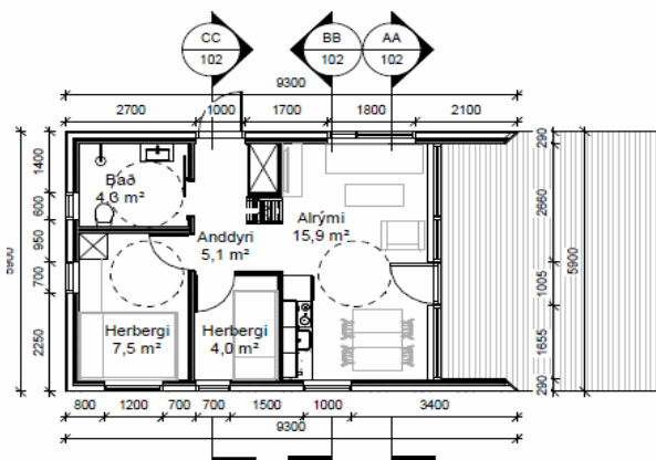
1 hæð 1 : 100
