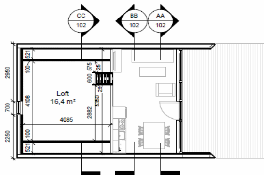
Loft 1 : 100
