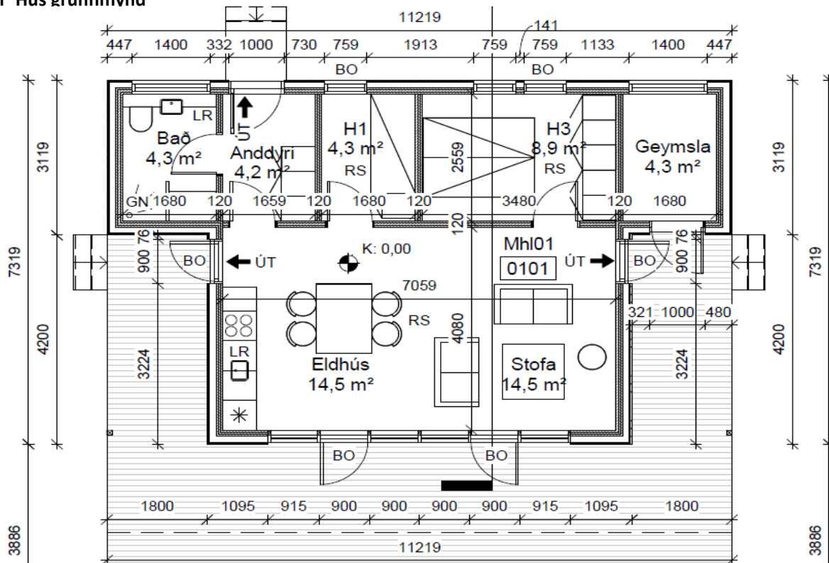
67m 2 Hús grunnmynd
